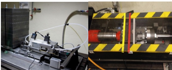
Banc à actionneurs parallèles (électrique-pneumatique) / banc ELEXC (hydraulique-électrique)
