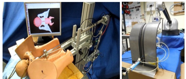
Simulateurs d'accouchement (BirthSim) et de péridurale (PeriSIM)
